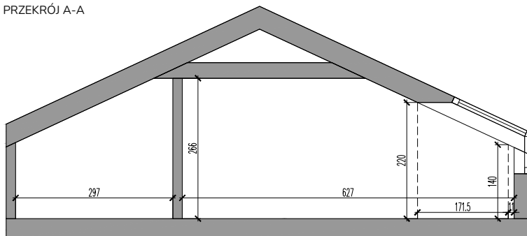
PRZEKRÓJ A-A
